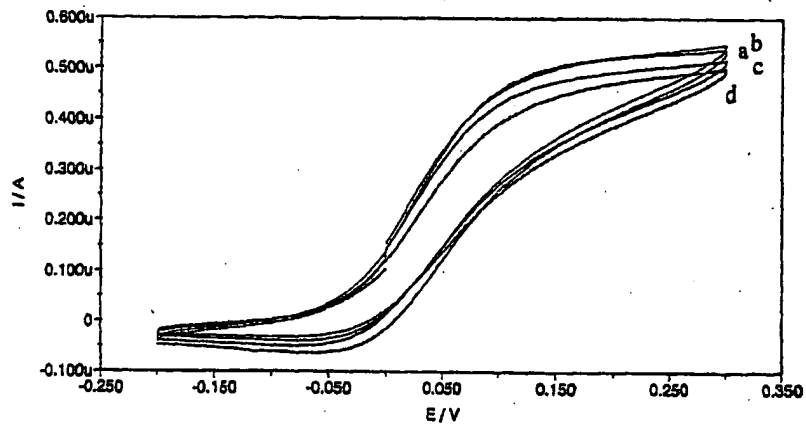
Abbildung 16: CV der TMPD-modifizierten Glukosebiosensoren mit Stärke-Schutzschicht, gemessen an unterschiedlichen Tagen, in gepufferter Glukoselösung, (pH 7.4 ; c_{(\text{Glukose})} 15 mM, c_{(\text{Cl}^-)} 154 mM), v = 50 \text{ mV/s} a: 1. Tag ; b: 9. Tag ; c: 18. Tag ; d: 46. Tag
